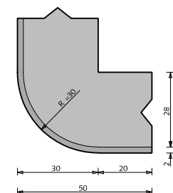
BOVENAANZICHT
